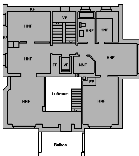
Grundriss 1. Obergeschoss:
