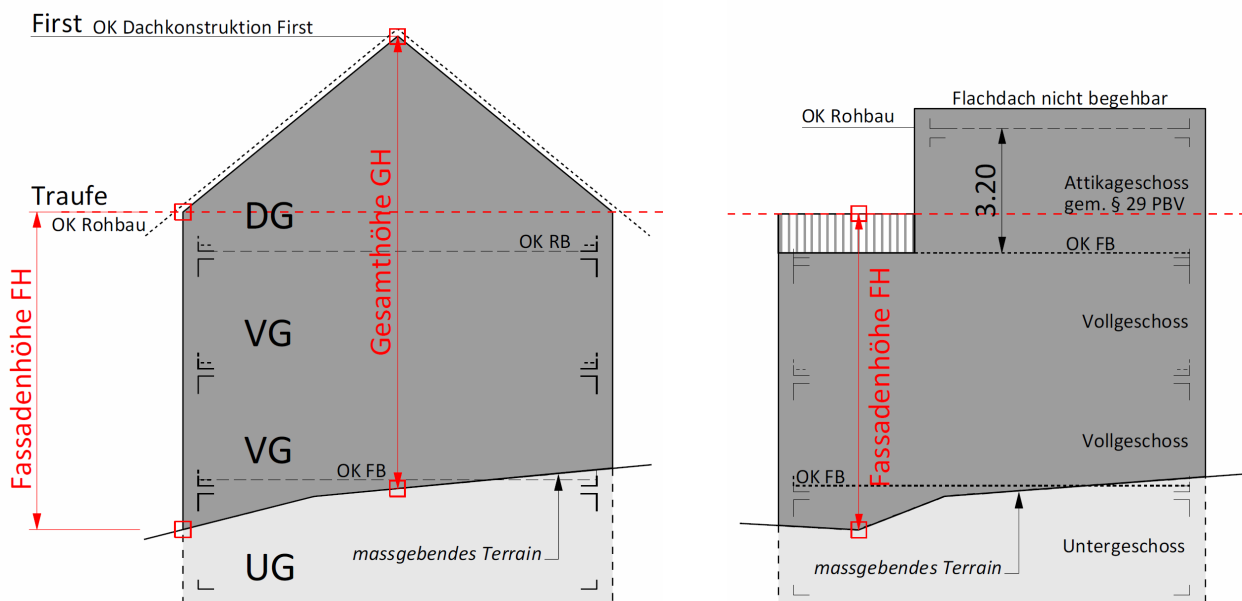
Schrägdach
